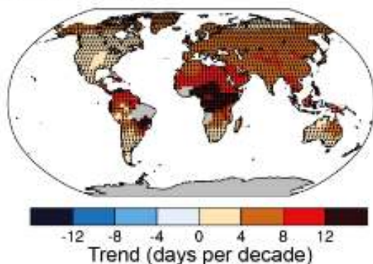
(d) Warm Days
